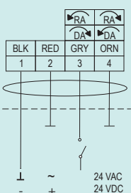
Commande TOUT OU RIEN, 2 fils
