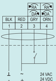
Ouvert / Fermé, Commande à 1 fil
