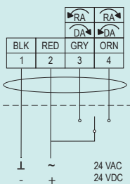
Commande à 3 points, 4 fils
