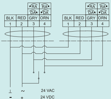
Commande à 3 points, Montage en parallèle, avec un transformateur
